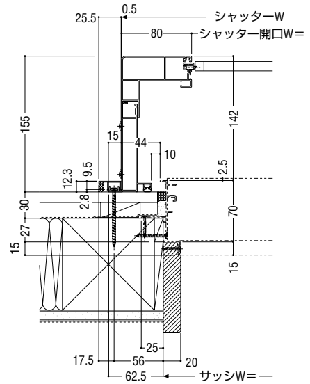
横断面
